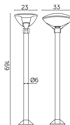
podstawa / base
